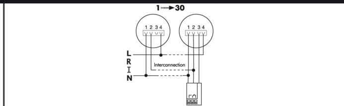
Tilsluttes 230 V AC og system + eksternt omskifterrelæ (tilhører) til tænd/sluk af eksterne apparater som f.eks. sirener, rotorblink og telefonomstillinger.
